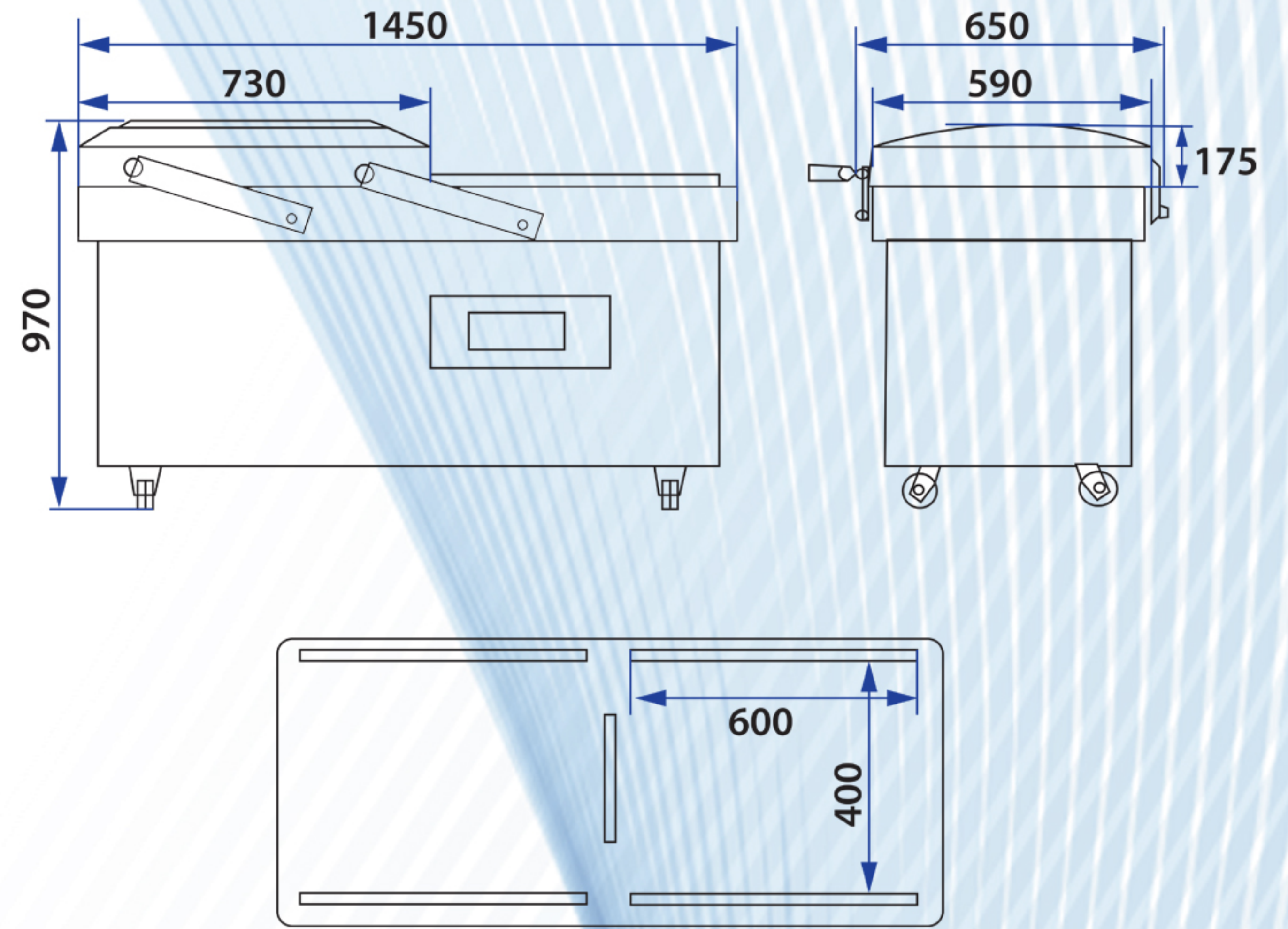
ขนาดตัวเครื่องซีลสุญญากาศ เบ็ลเทอร์ 24 BELTER-24 MACHINE DIMENSION
