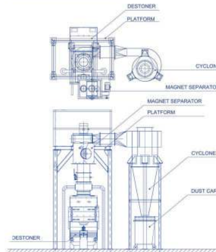
ภาพแสดงตำแหน่งการติดตั้งเครื่องคัดแยกหิน และเครื่องตรวจจับโลหะ
